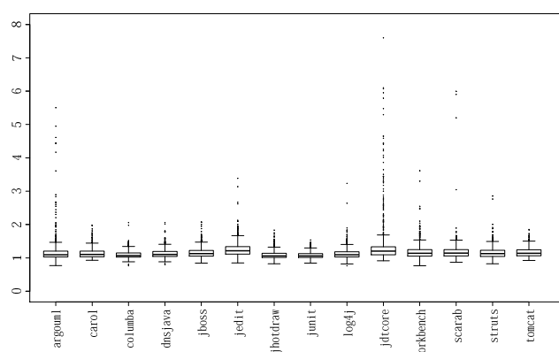
図 9: 全ての変更に対する実行時間の比較
