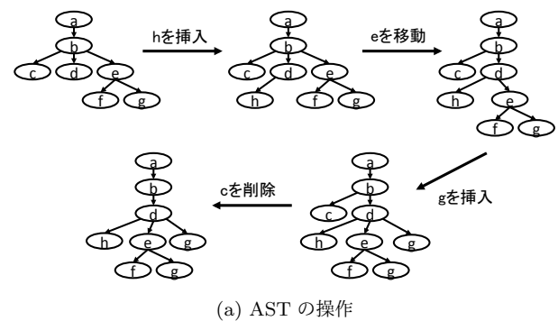
(a) AST の操作
