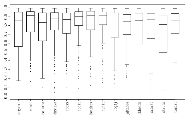
図 8: 編集スクリプトの長さが異なる変更における長さの比較
