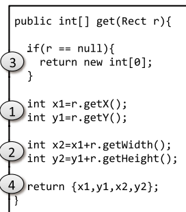
図 6 コードの記述順序の例 Fig. 6 An example of code writing order.
