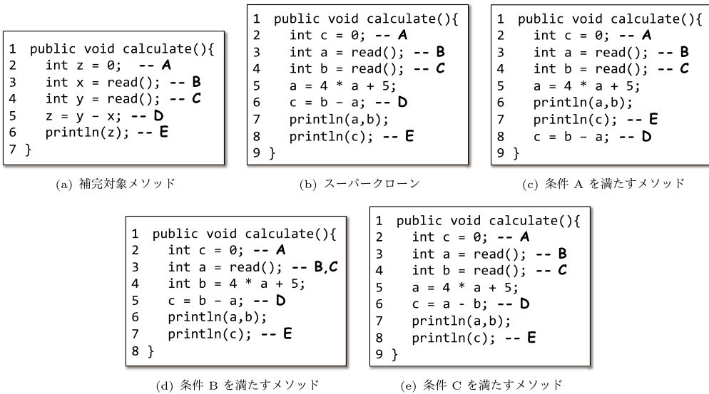
図 5 補完対象メソッド，スーパークローン，及びスーパークローンにならないメソッドの例 ((b) から (e) は補完候補データベースに登録されているメソッドである)
