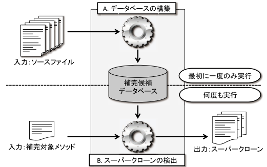
図 3 補完候補の有無を判定する方法の概要
