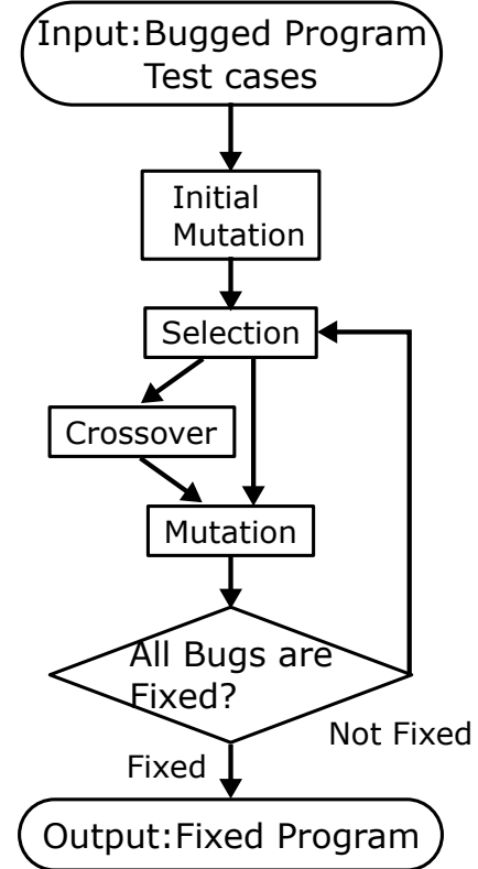
Fig. 1. Abstract of GenProg
