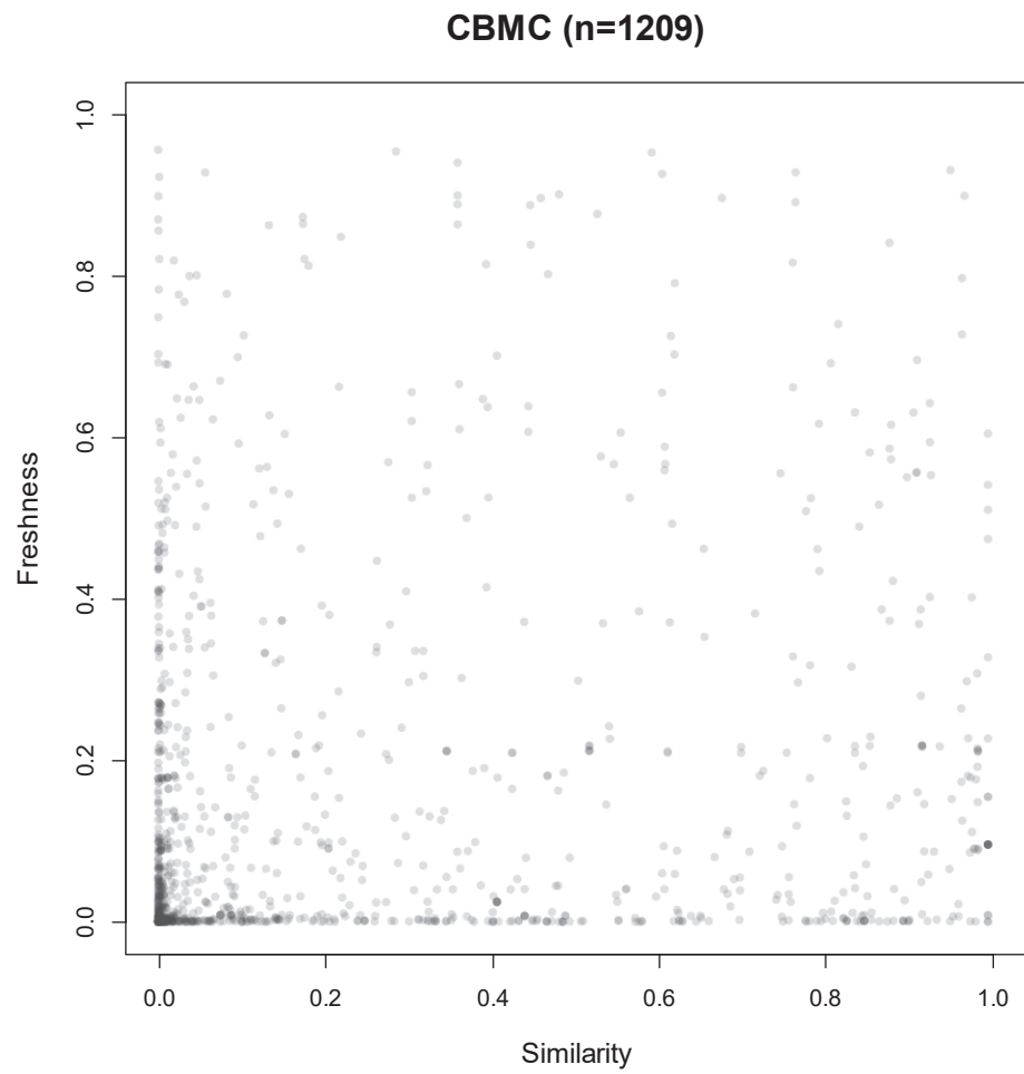
図 7: 更新順と類似度順の関係 (CBMC)
