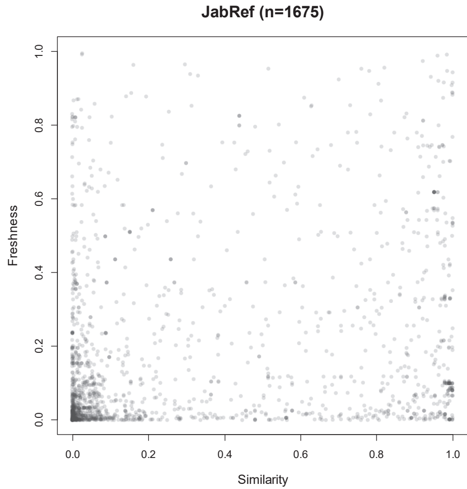
図 9: 更新順と類似度順の関係 (JabRef)
