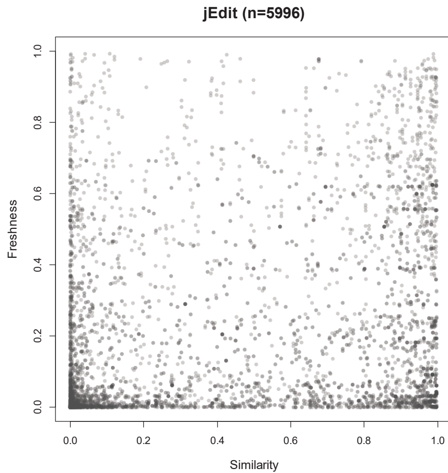
図 11: 更新順と類似度順の関係 (jEdit)
