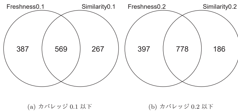
図 10: 各基準でカバレッジの小さい挿入行の集合によるベン図 (JabRef)
