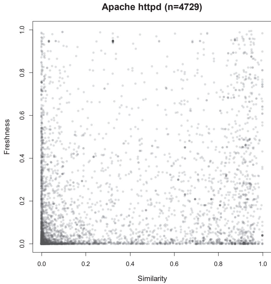
図 5: 更新順と類似度順の関係 (Apache httpd)
