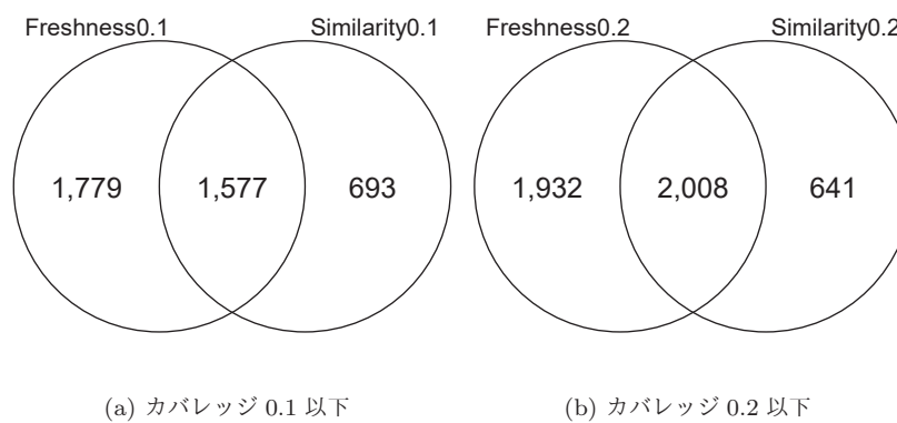
図 12: 各基準でカバレッジの小さい挿入行の集合によるベン図 (jEdit)
