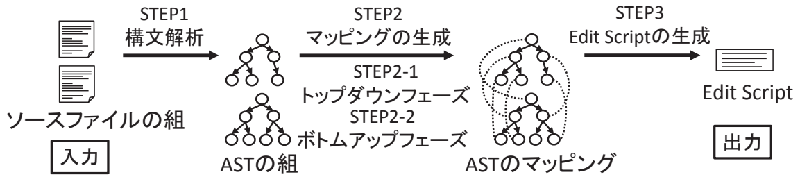
図 7: GumTree の概要
