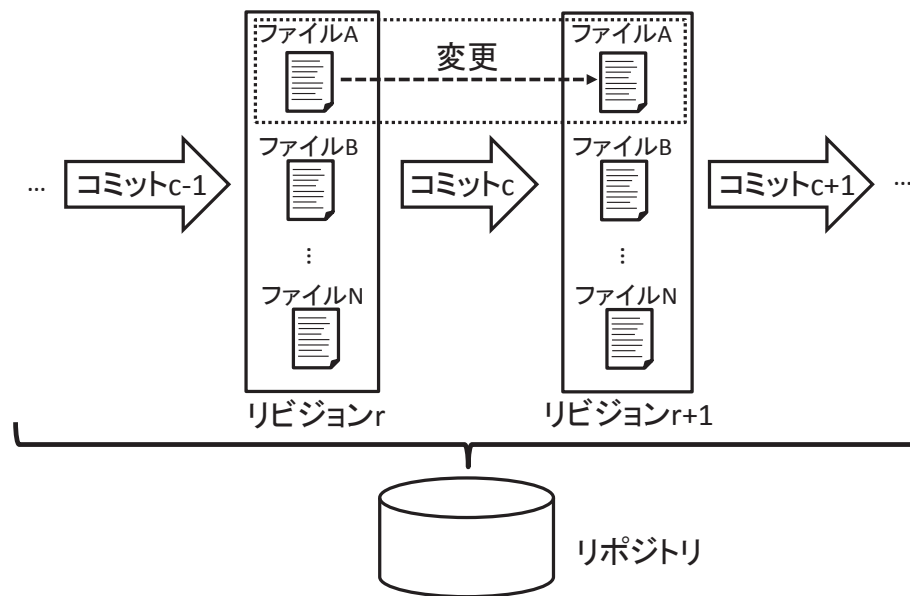
図 15: リポジトリからの変更の取得
