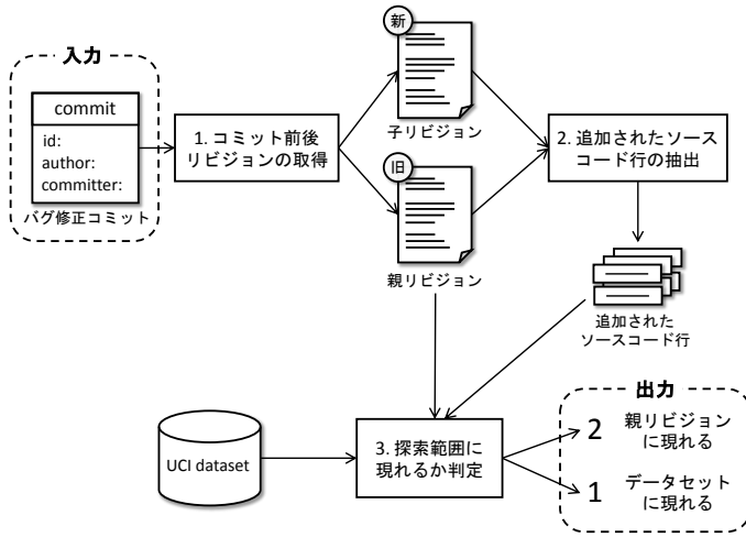
図 2 実験 1, 実験 2 の流れ
