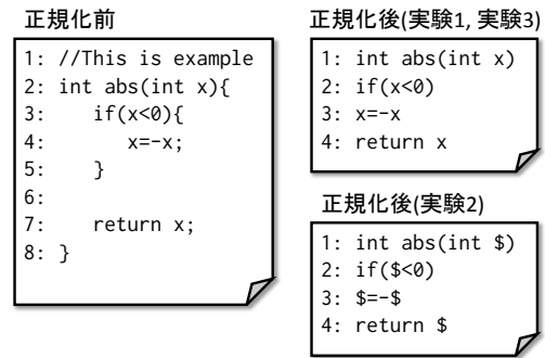
図 3 正規化の流れ
