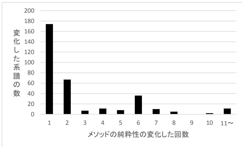
図 9: jEdit におけるメソッドの純粋性が変化した回数
