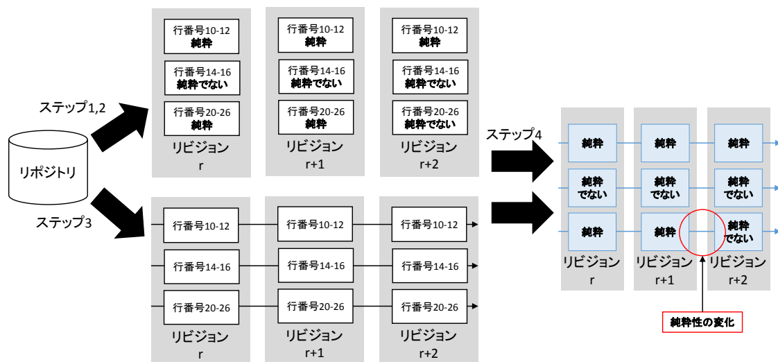
図 4: 純粋性の変化を検出する手法の概要
