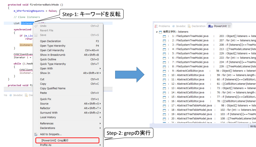
図 1: PowerUnit の使用例
