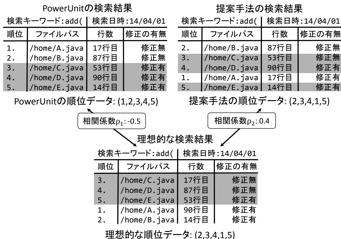
図 8: 順位データの例
