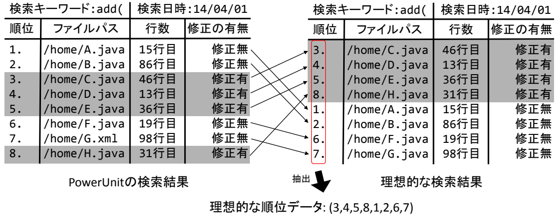
図 7: 理想的な順位データの生成例
