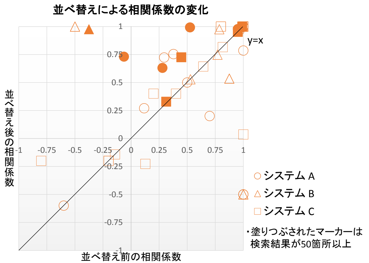
図 9: 並べ替えによる相関係数の変化
