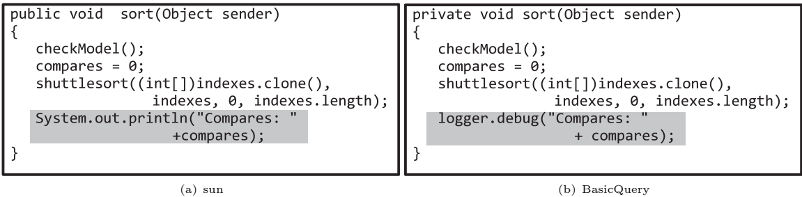
図 8 ライブラリ化すべきと判断したコードクローンの例 Fig. 8 An instance of method cloneset suite for library building.
