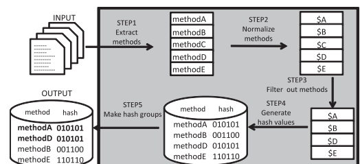
図1 石原らの手法の概要
