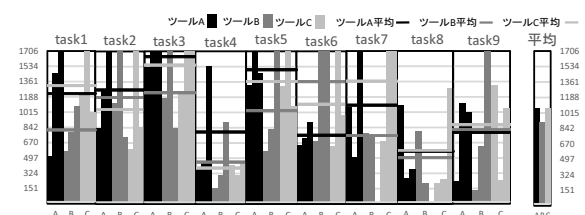
図7 所要時間
