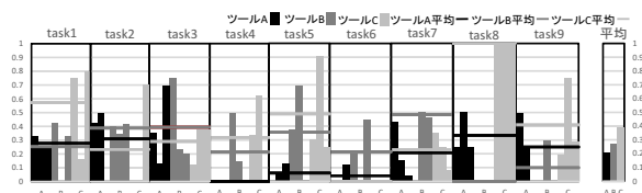
図6 貢献率
