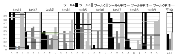
図5 利用率
