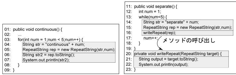
(a) 1つのメソッドで実装した例（委譲なし）
