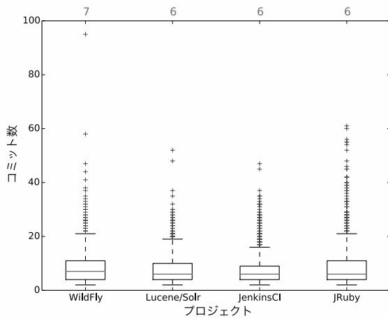
図 4: 各クラスタのコミット数分布
