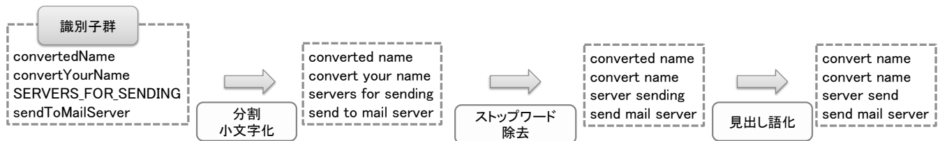
図 2: 識別子の英単語の見出し語化までの過程
