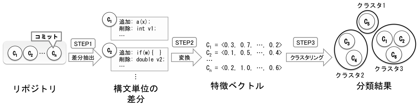
図 1: コミット分類の流れ
