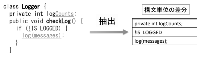
図 3: ソースコード変更と構文単位の差分の例
