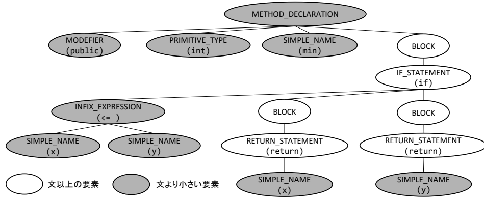
図 2 抽象構文木
