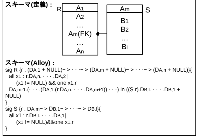
図 5 スキーマのAlloyへの変換
