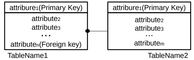
図 1 スキーマ例
