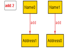
図 1 スキーマ例
