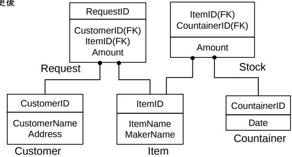
図 10 検証対象のスキーマ
