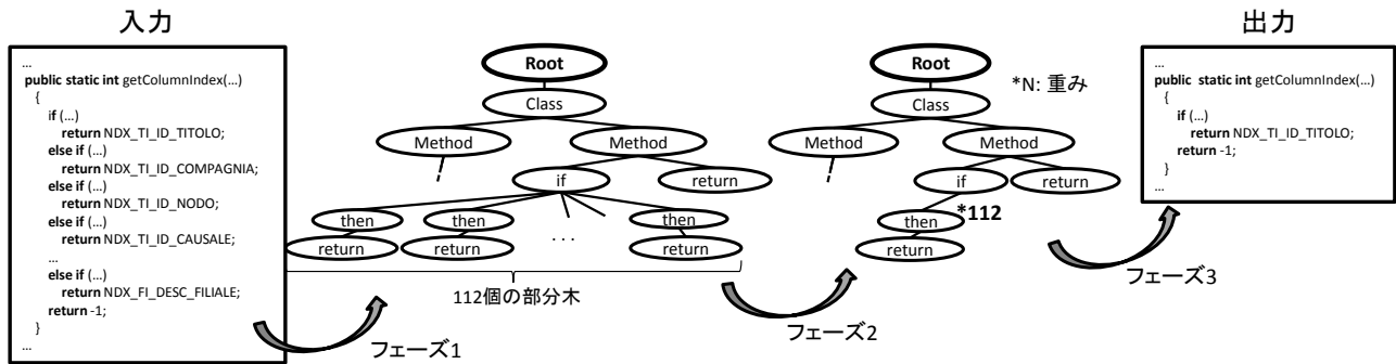
図 2 図 1(b) のソースコードに対する提案手法の流れ Fig. 2 Proposed Method for Fig.1(b)
