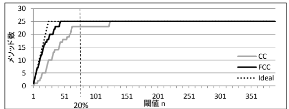
(a) サイクロマチック数
