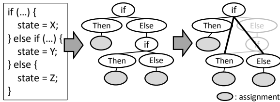
図 3 else-if 節の変形 Fig. 3 Transformation of else-if Statements
