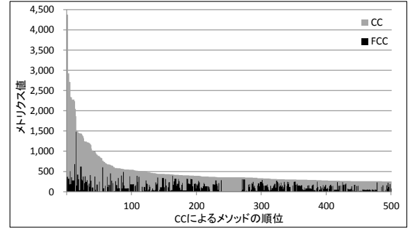
(a) サイクロマチック数
