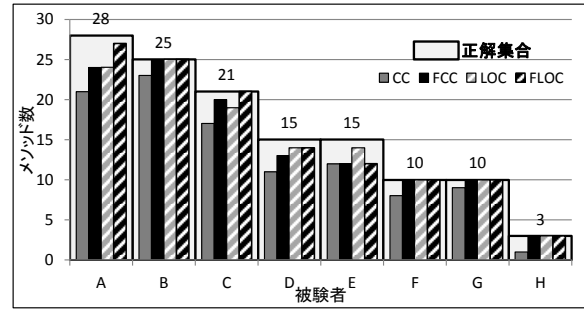
図 7 上位 20 パーセント中の複雑なメソッド検出数
