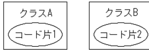
図 6: DCH=\infty
