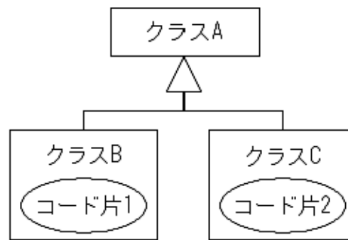
図 5: DCH=1
