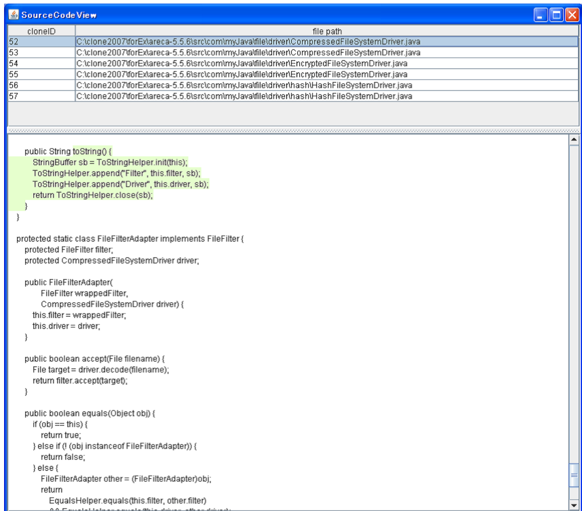
図 9: DCHchecker の SourceCodeView
