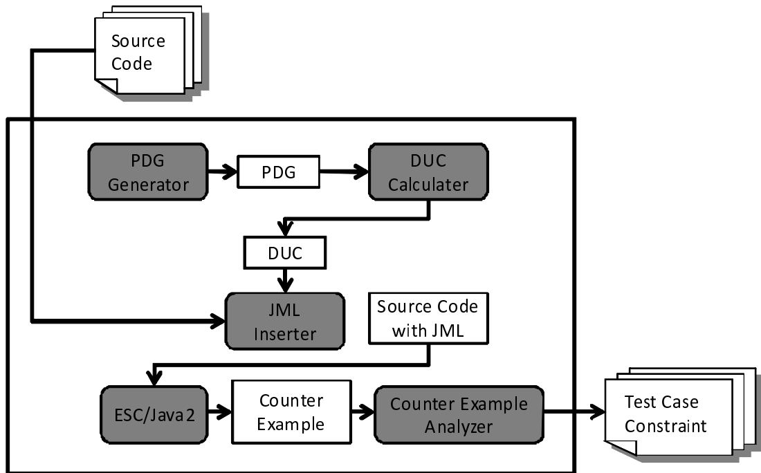
図 5: 既存手法による処理の概要
