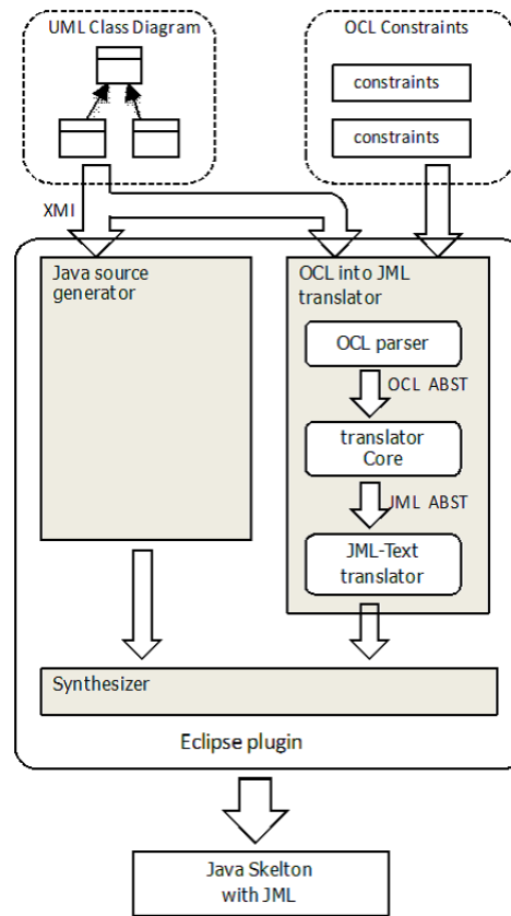
図 7: ツール全体図
