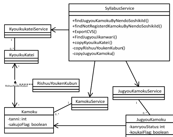
図 5 教務システムの Service クラスの一部
