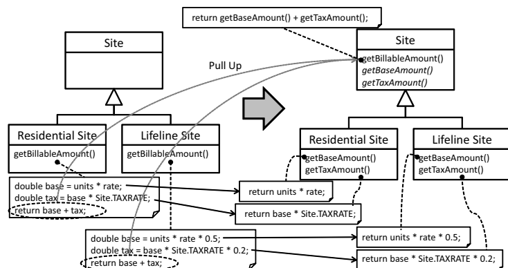
図 1 Template Method パターンの適用例
